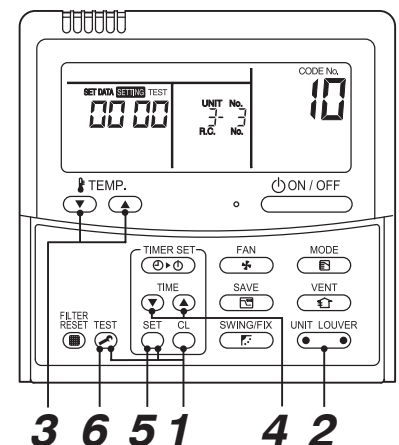
<Fig. 1 RBC-AMT32E>
